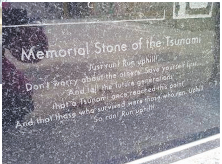
海嘯紀念碑
